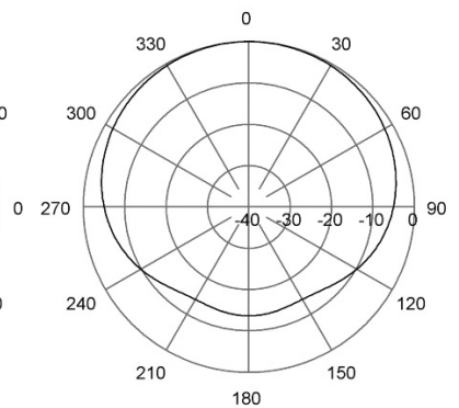
H-Plane | 400 MHz
