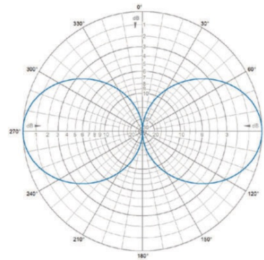
E-Plane | 445 MHz
